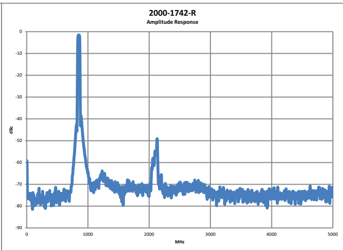
Stopband
