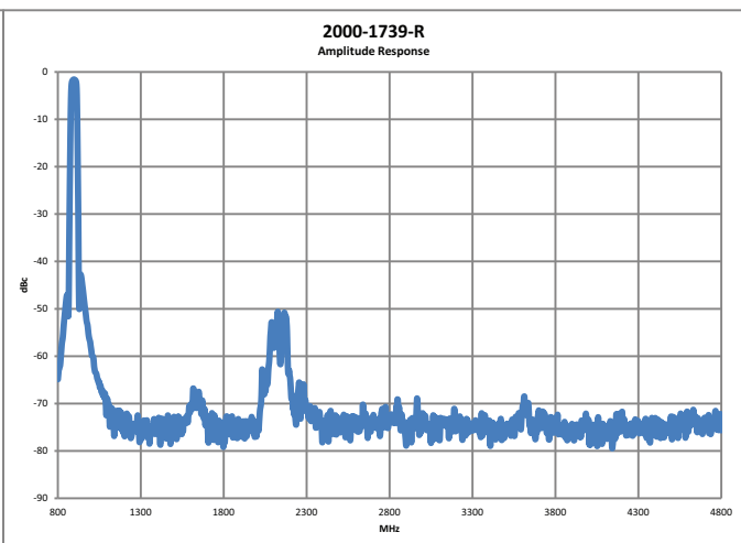
Stopband
