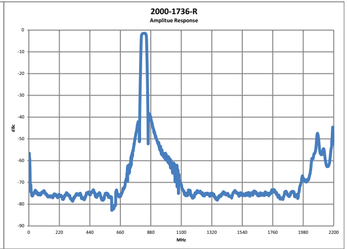
Stopband
