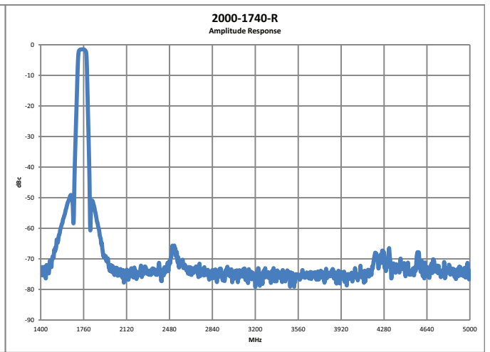
Stopband
